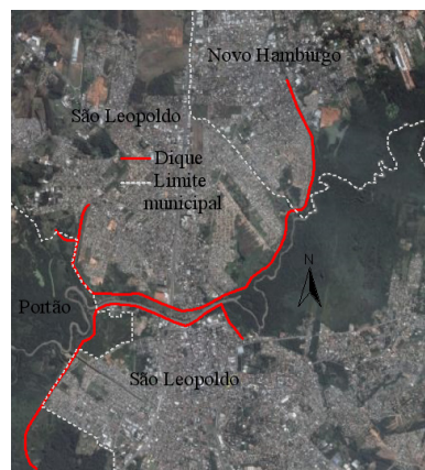
Fig. 2 - Vista aérea dos pôlderes IV e V do SCEVRS.
