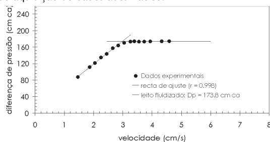
Fig. 9 - Influência da velocidade do fluido na queda de pressão do leito.
