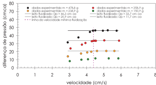
Fig. 8 - Velocidade mínima de fluidização diferentes alturas de areia.
