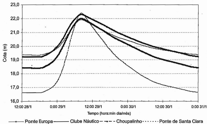
Figura 19 - Níveis de água obtidos através de simulação numérica.
