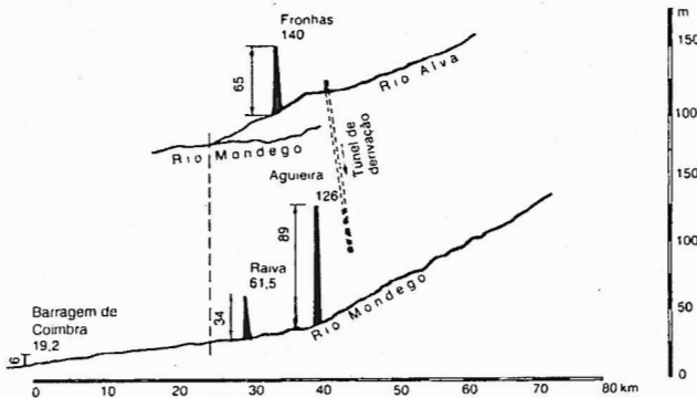
Figura 3 - Esquemática do Aproveitamento Hidráulico do Mondego.
