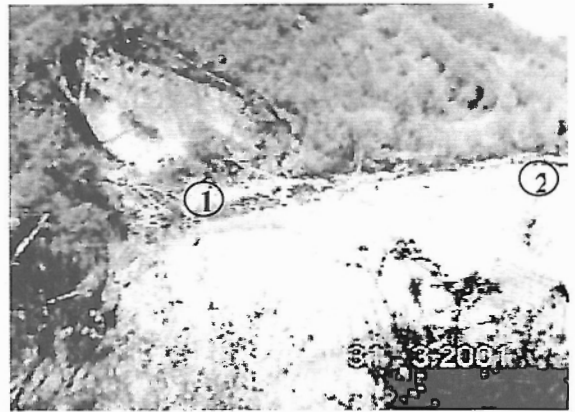
Foto 14 - Chã (Cinfães, rio Bestança, margem sul do rio Douro). 1. Parte da acumulação resultante do deslizamento que constituiu a barragem natural. 2. Parte da área erodida pela destruição da barragem natural.
