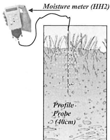
Figura 3 Equipamento utilizado na monitorização da humidade do solo.
