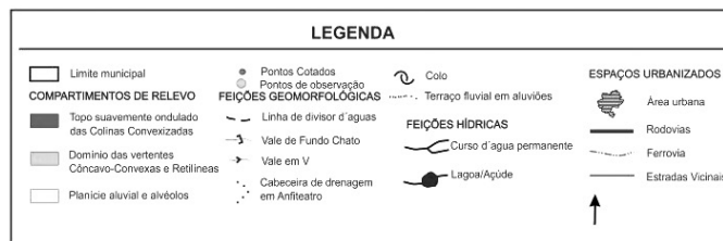
Figura 6 Pontos de observação com cabeceira de drenagem em formato de anfiteatro. Fonte: Felipe (2015).
