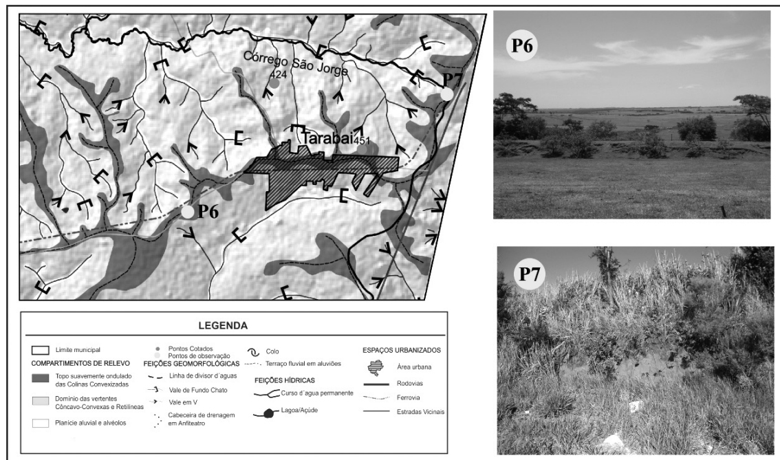
Figura 8 Pontos de observação com topos estreitos alongados. Fonte: Felipe (2015).
