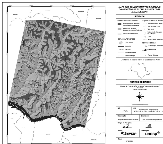
Figura 5 Mapa dos compartimentos de relevo do município de Estrela do Norte-SP e adjacências. Fonte: Felipe (2015).
