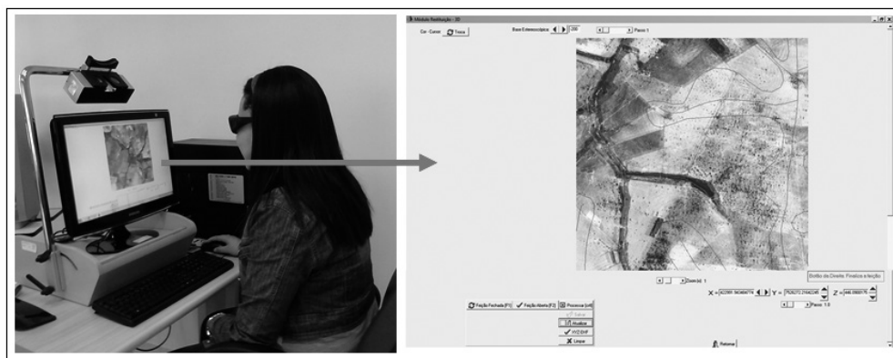
Figura 3 Extração das feições geomorfológicas a partir do método anaglifo. Fonte: Felipe (2015)
