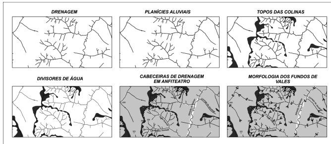
Figura 4 Vetorização das feições geomorfológicas. Fonte: Felipe (2015).
