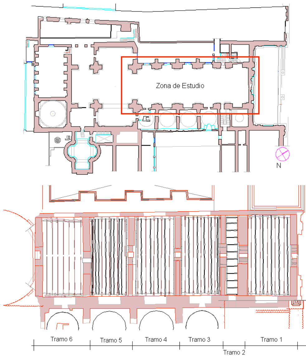
Fig. 3. Planta de la iglesia de San Ignacio
